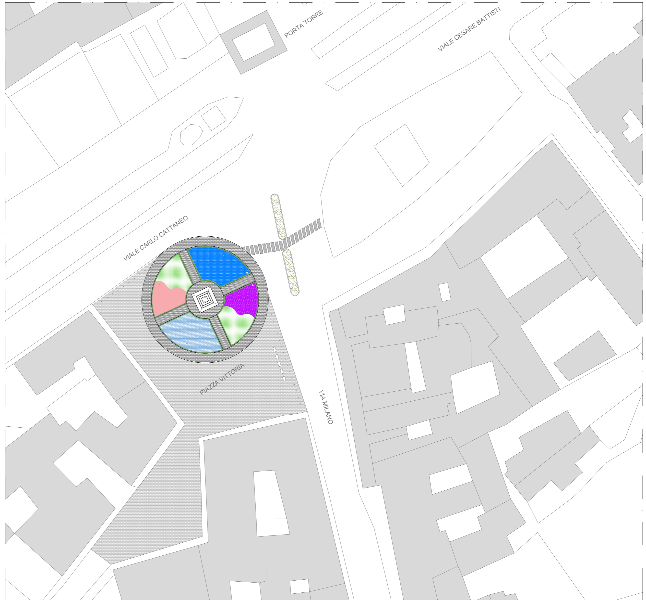
INQUADRAMENTO PLANIMETRICO 1:500
